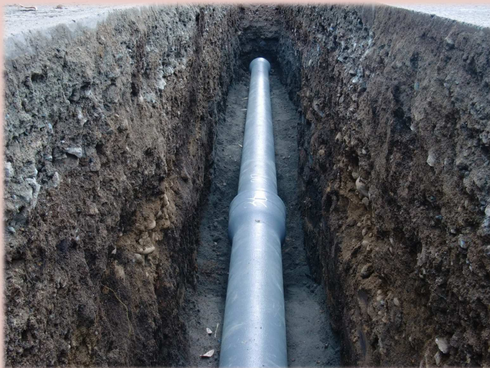
耐震管(ダクタイル鋳鉄管 GX 形)の布設工事
