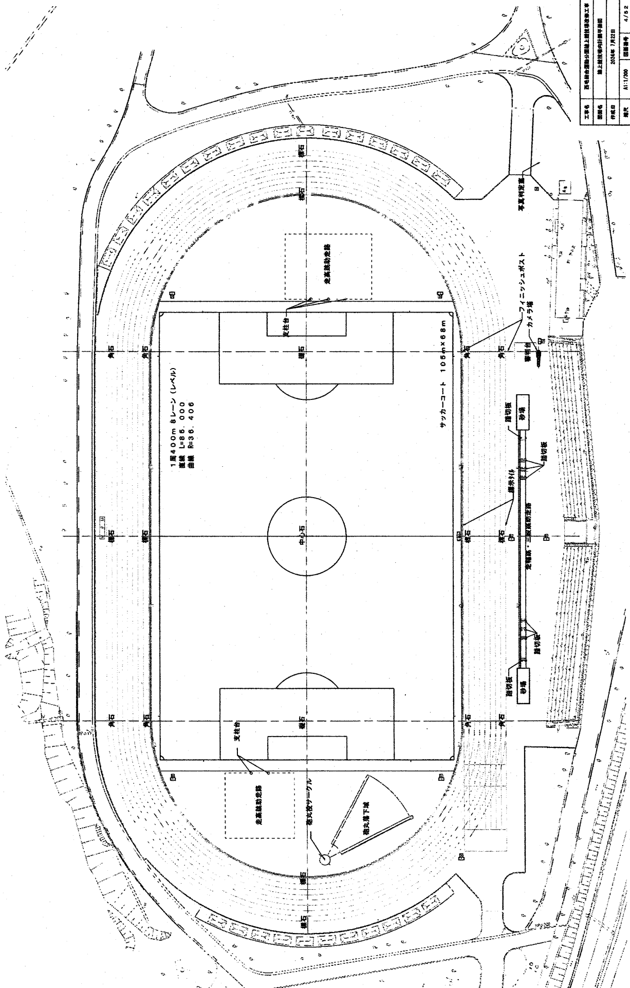
陸上競技場内計画平面図
