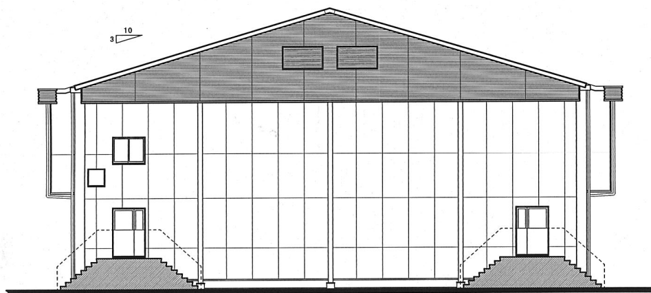
東 立 面 図 (現 況) S=1:100
