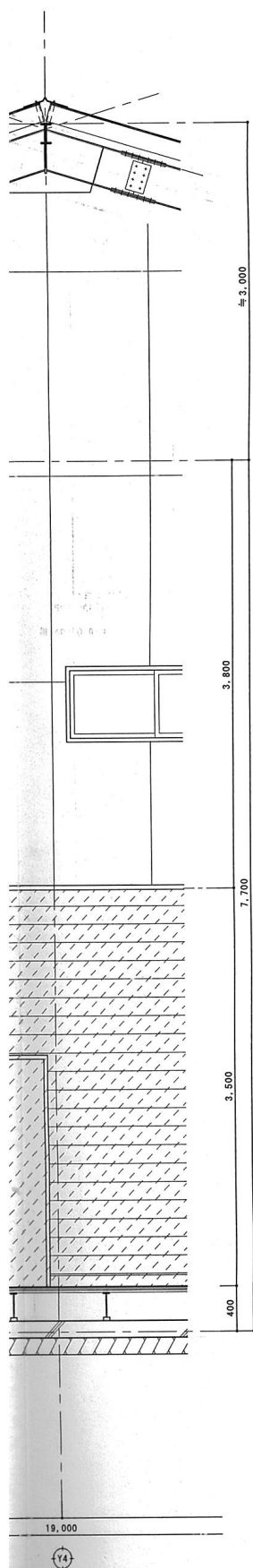
矩計図 S=1:30
