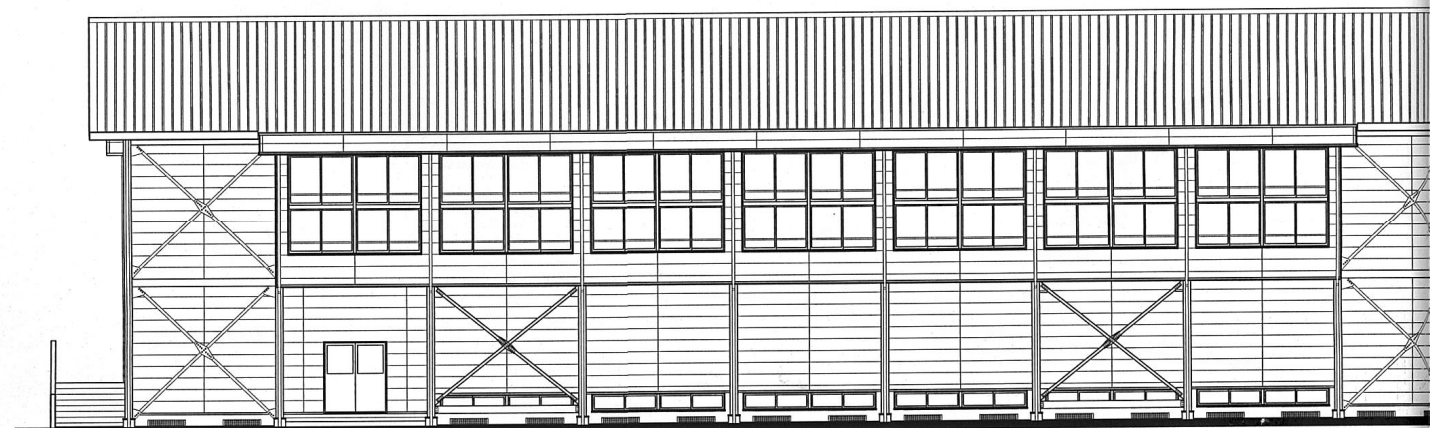
北 立 面 図 (実 施) S=1:100
