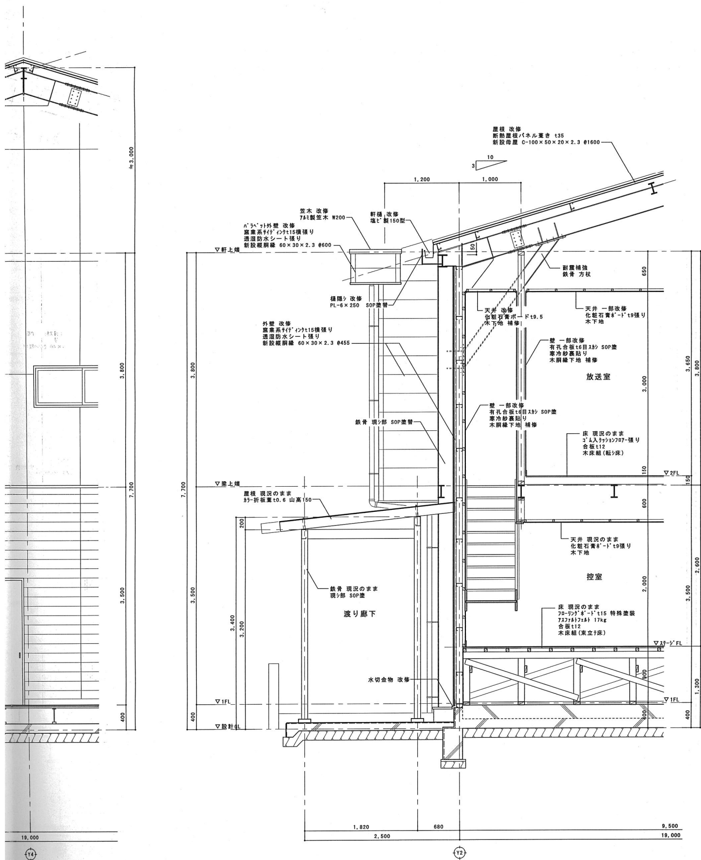
矩計図 S=1:30
