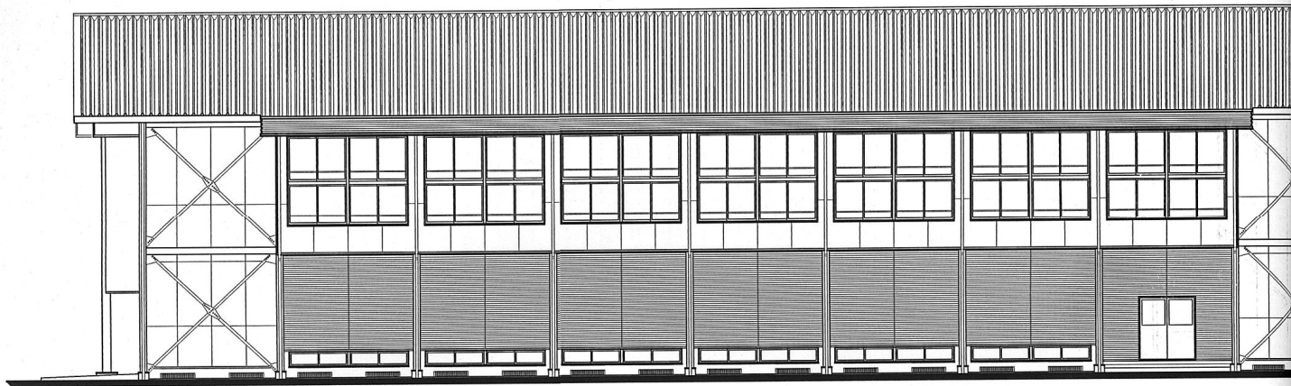
南 立 面 図 (現 況) S=1:100
