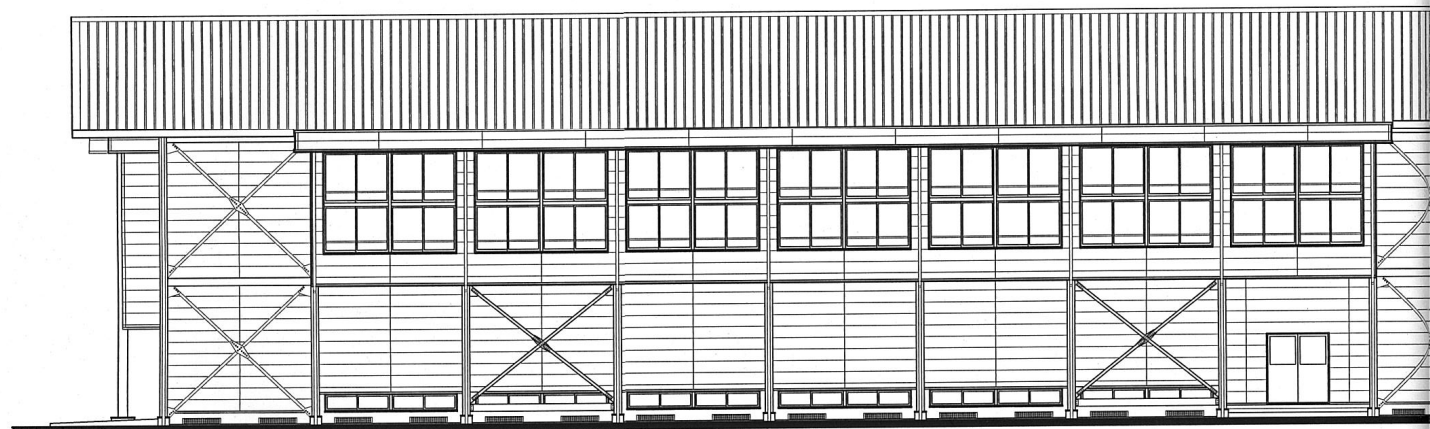
南 立 面 図 (実 施) S=1:100
