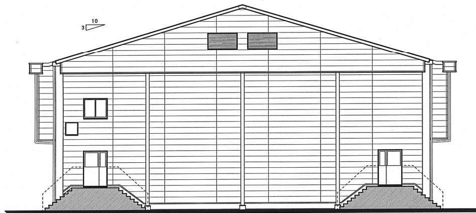
東 立 面 図 (実 施) S=1:100
