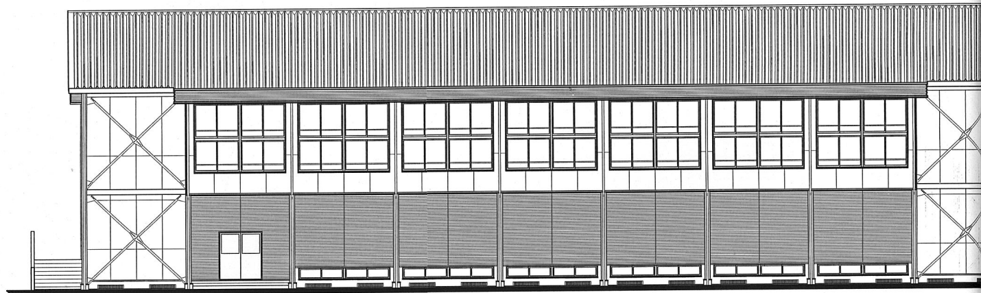
北 立 面 図 (現 況) S=1:100
