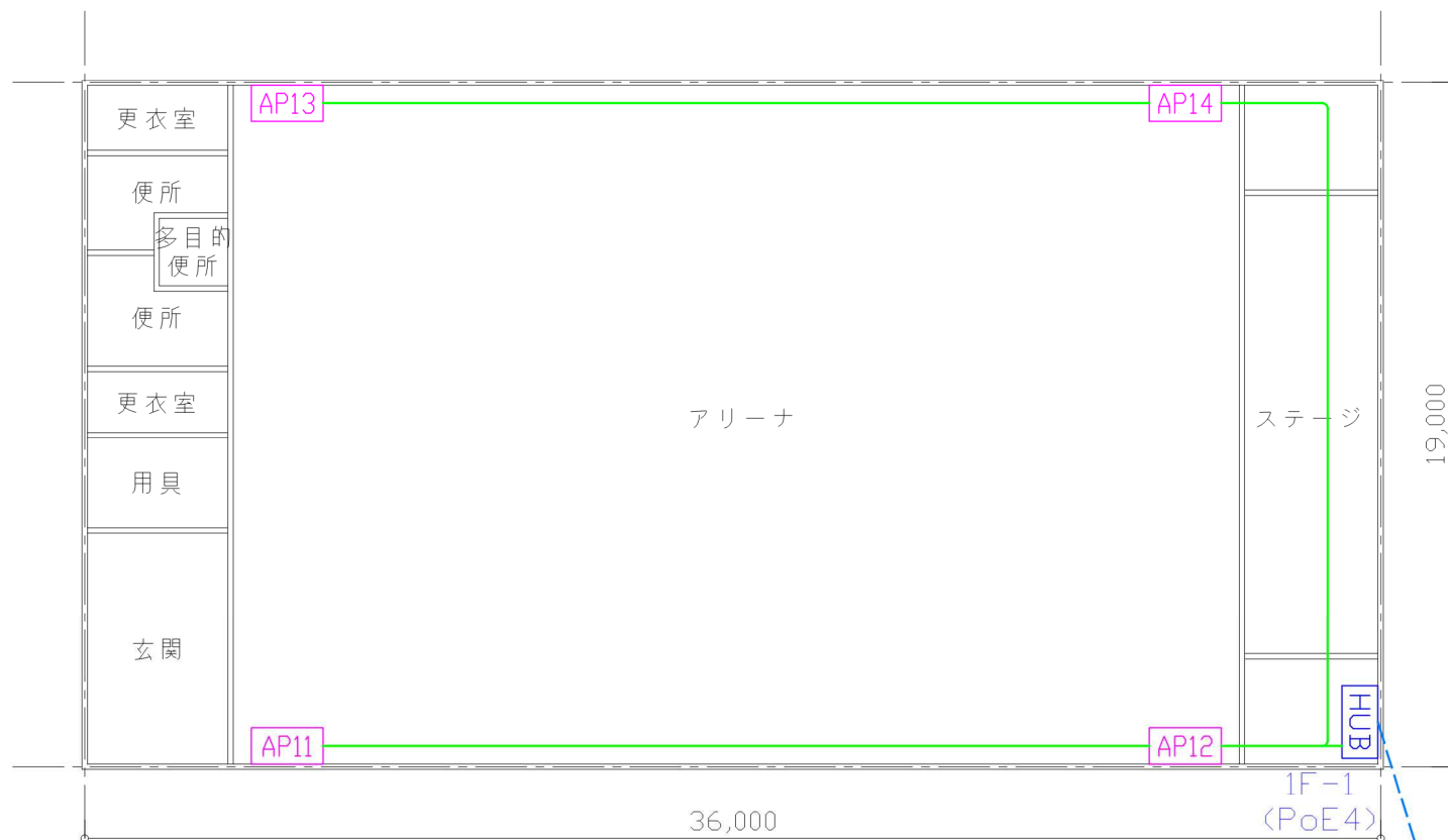
1 階平面図
