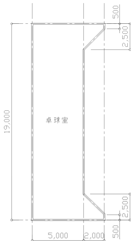
2 階平面図
