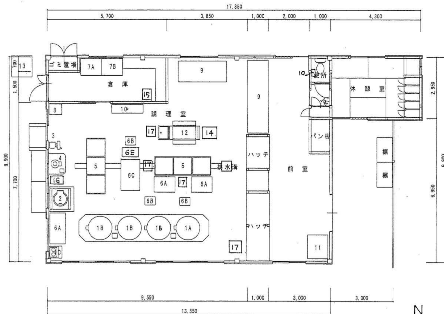
碓東小学校給食室 機器平面図 S=1:100
