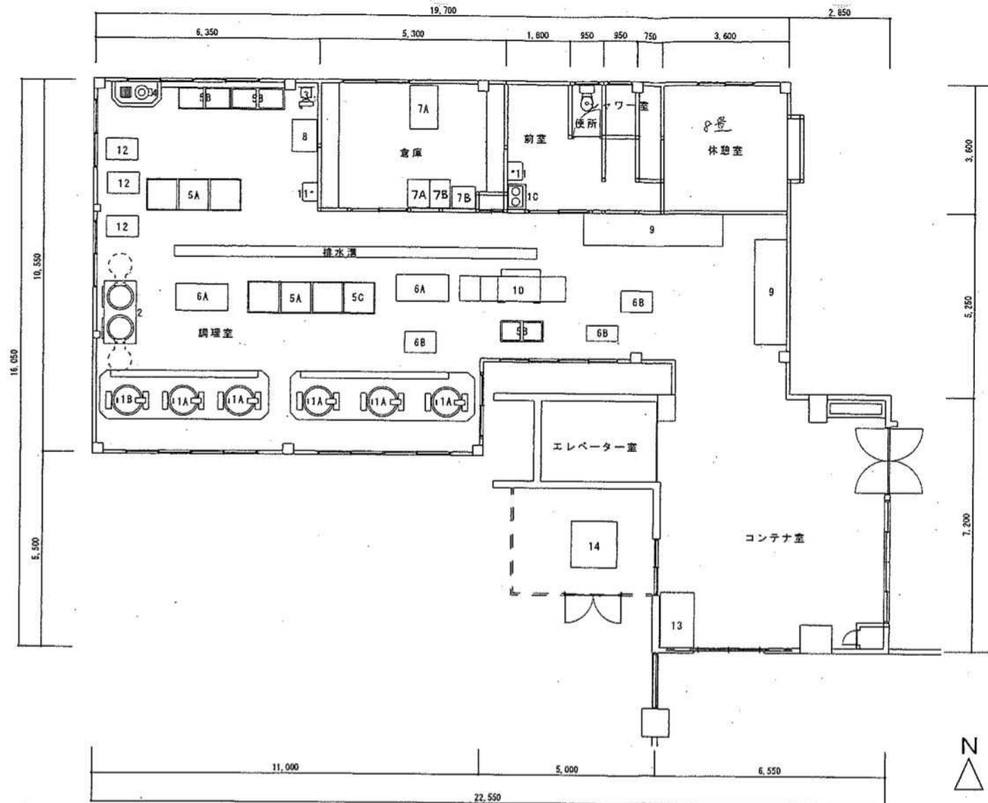
第一中学校給食室 機器平面図 S=1:100
