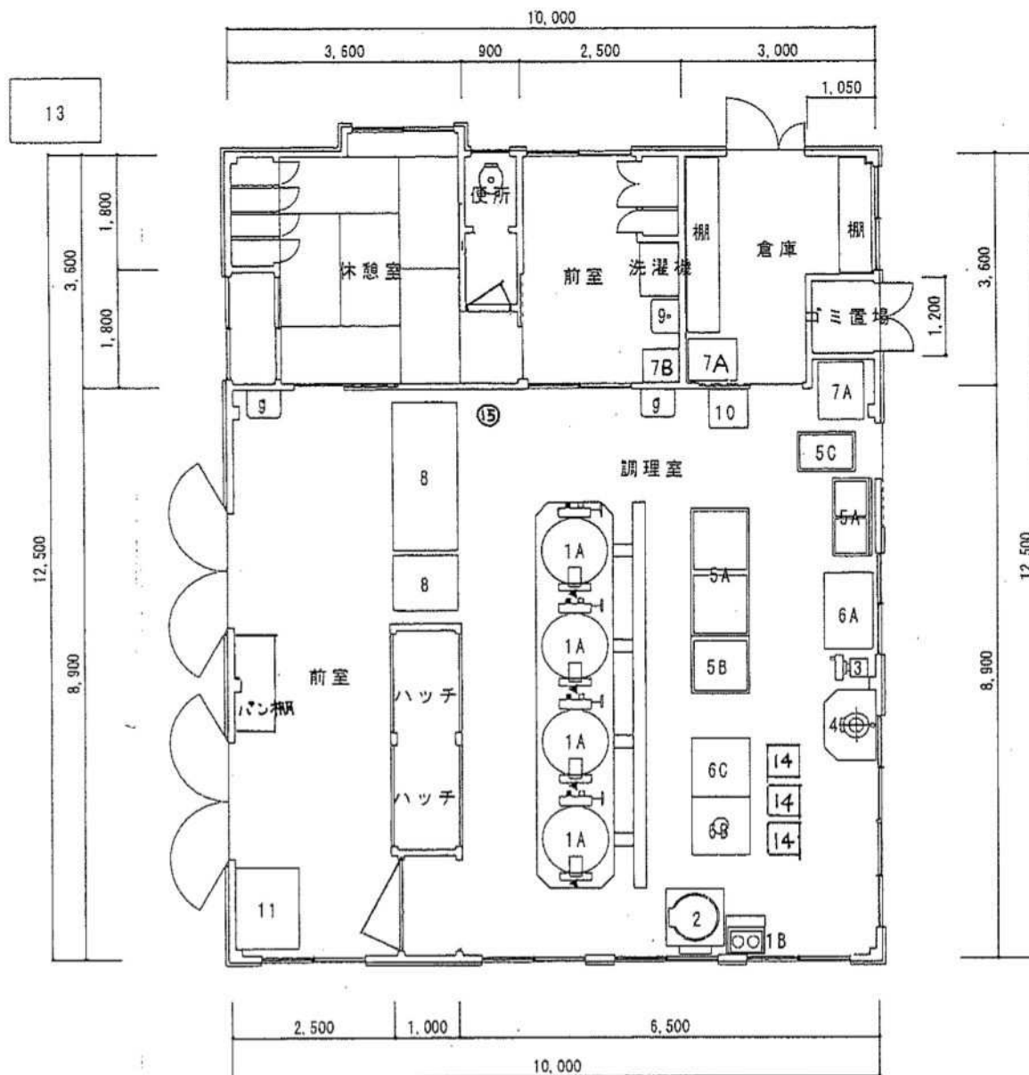
磯部小学校給食室 機器平面図 S=1:100
