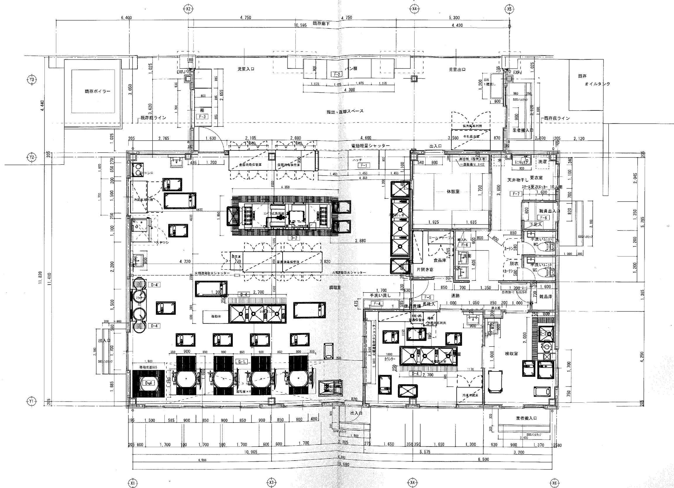
平面詳細図 1/50
