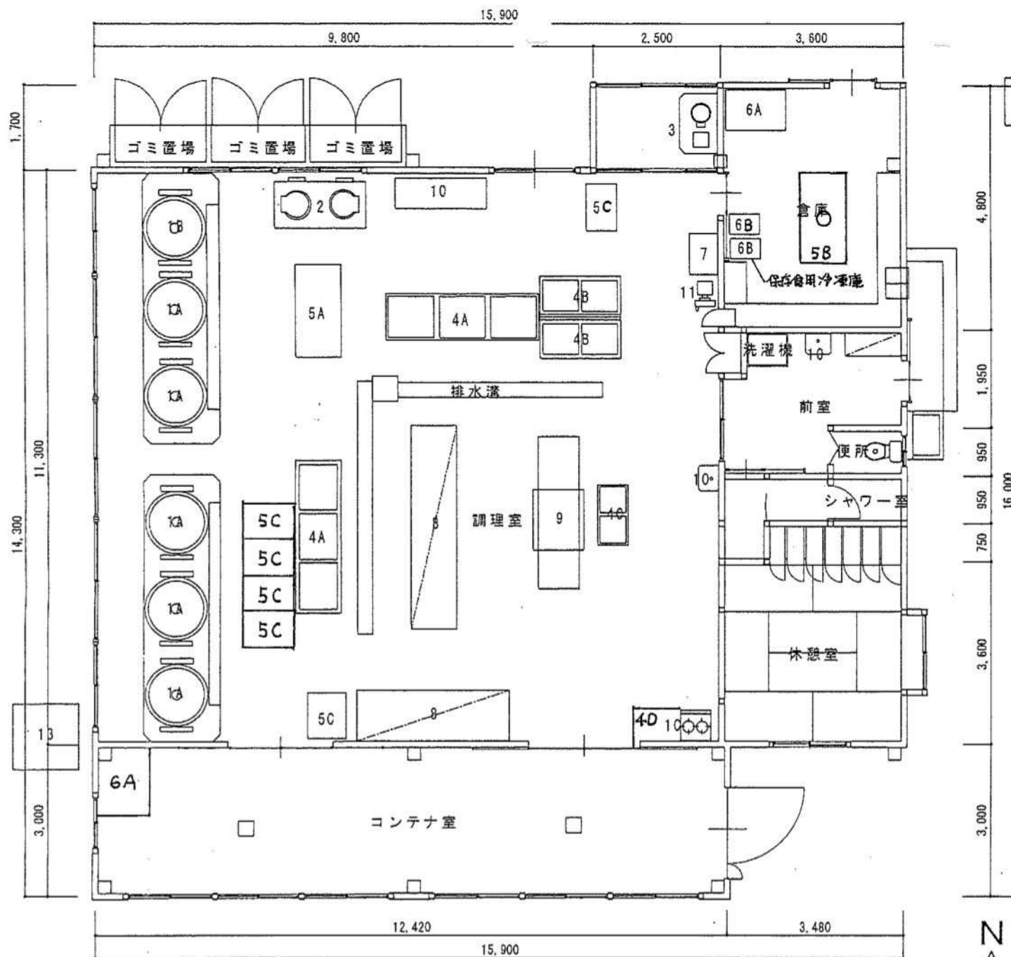
第二中学校給食室 機器平面図 S=1:100
