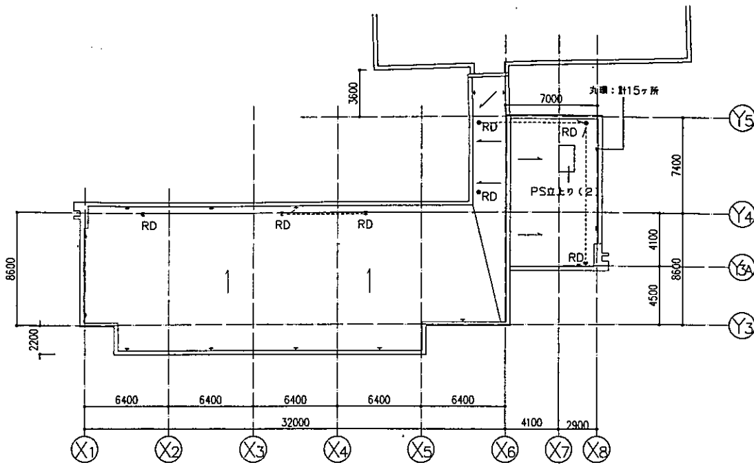
屋根伏図 1/200
