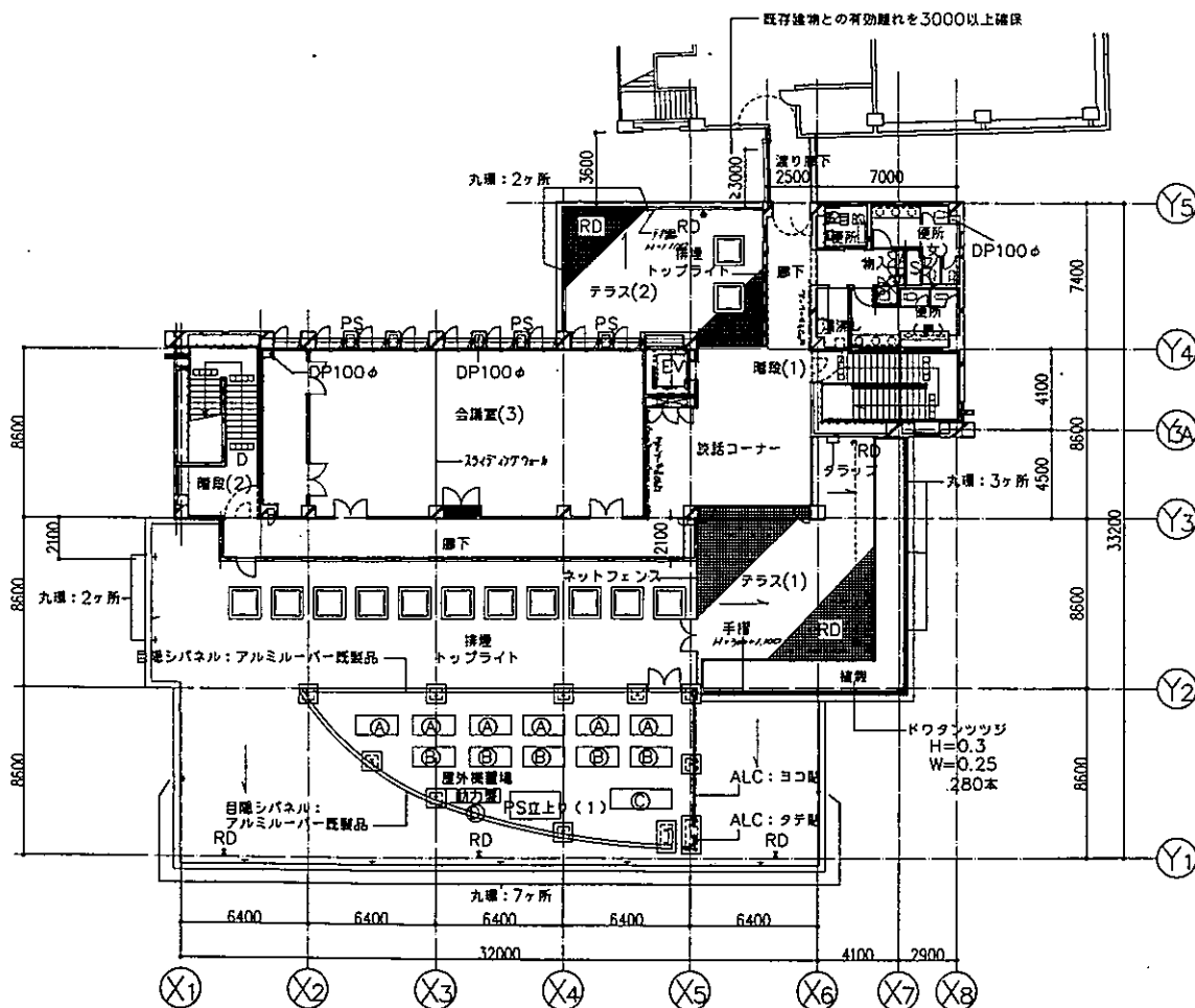
3階平面図 1/200
