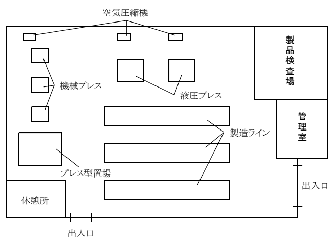
工場内の配置図
