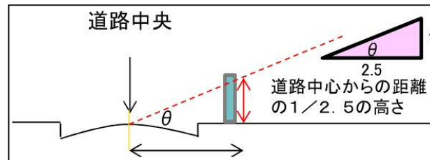
図2-3 通行障害建築物の対象とすることが可能になったブロック塀等
