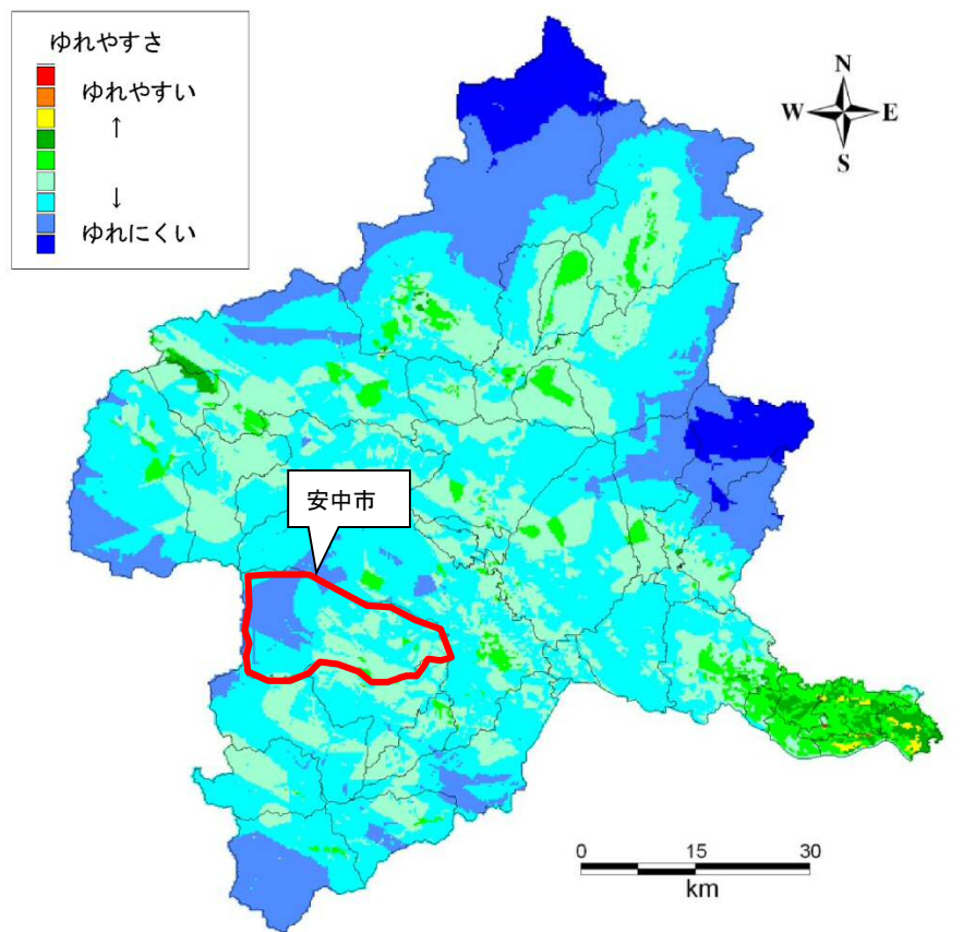
図1-4 予防対策用に設定した各市町村直下の地震による揺れやすさの分布
