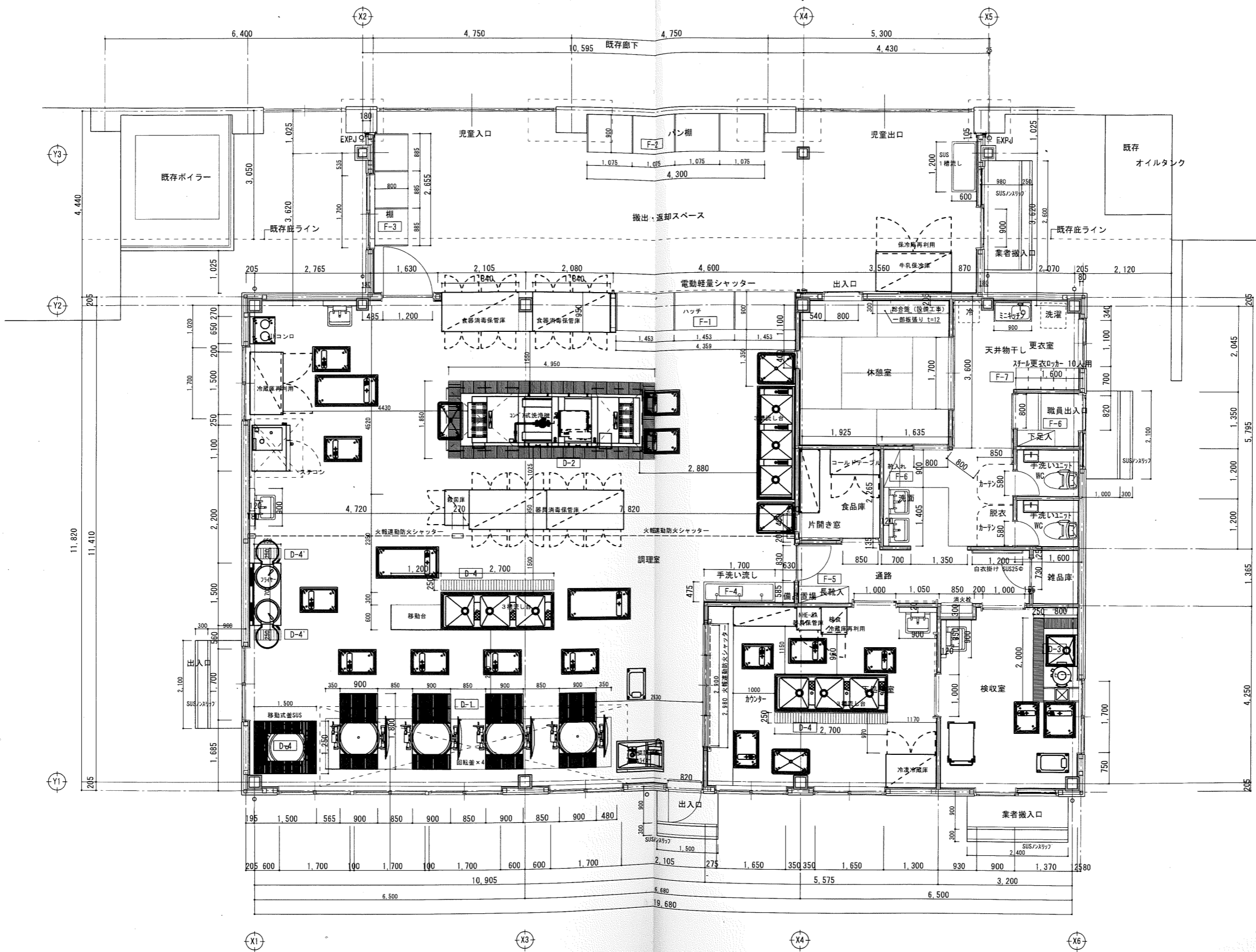
平面詳細図 1/50
